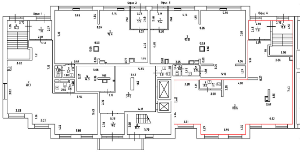
1-й этаж
